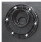
Рис. 5 Поворотный диск в сборе с неподвижным диском и саморезами
