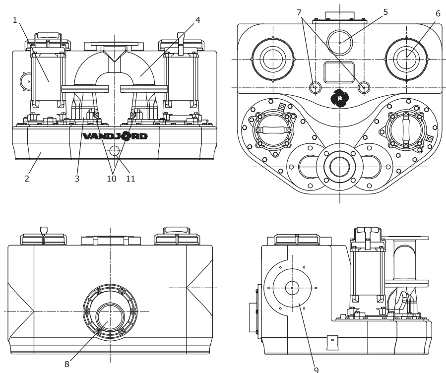
Рис. 1 Компоненты установки Prolift
