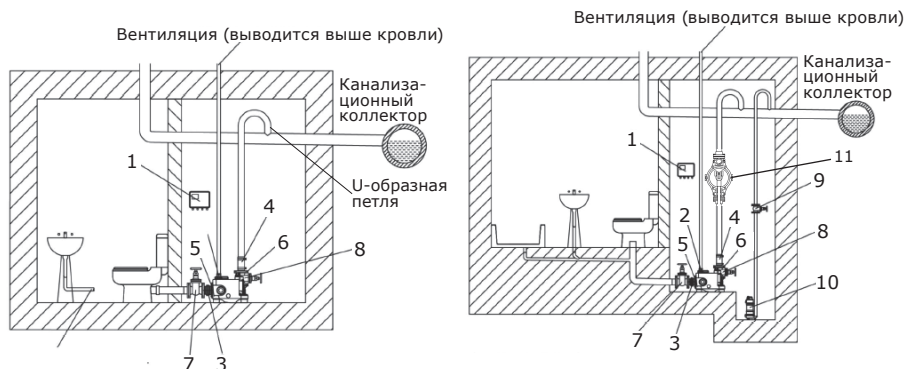
Рис. 2 Схема монтажа с прямым подключением (слева) и в приямке (справа)
